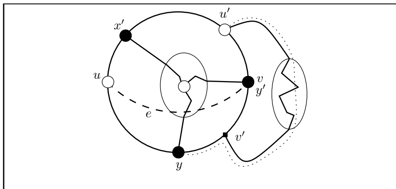
Joonis 10.21. Variant 2.1.2: \bar{K}_{3,3}
