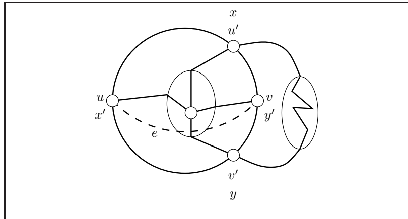
Joonis 10.23. Variant 2.2.2, esimene võimalus: K_5
