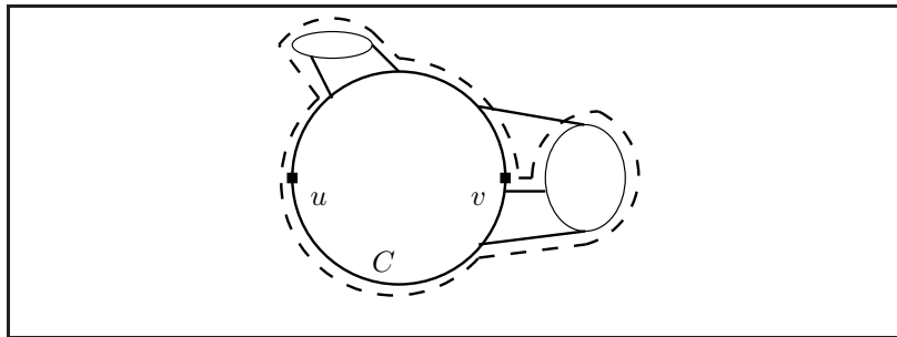
Joonis 10.12. Tsükkel üle välimiste komponentide
