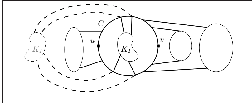
Joonis 10.14. Komponenti K_I tsüklilt väljaviimine
