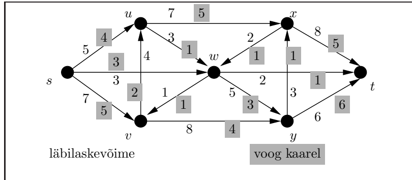
Joonis 6.1. Näide võrgust ja voost temas
