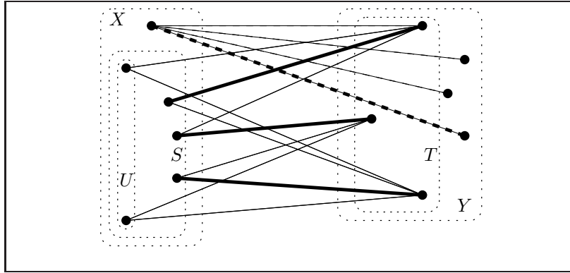
Joonis 7.3. Tekkivad hulgad Königi teoreemi tõestuses
