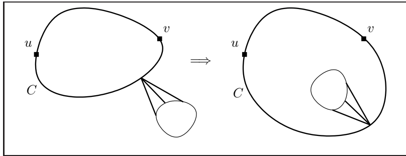
Joonis 10.11. Ühes tippu kinnituv komponent tsükli C sisse
