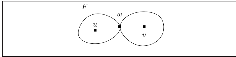
Joonis 10.4. Tipp w eraldab tippu u ja v
