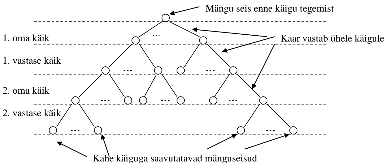
Joonis 1. Käikude planeerimispuu
